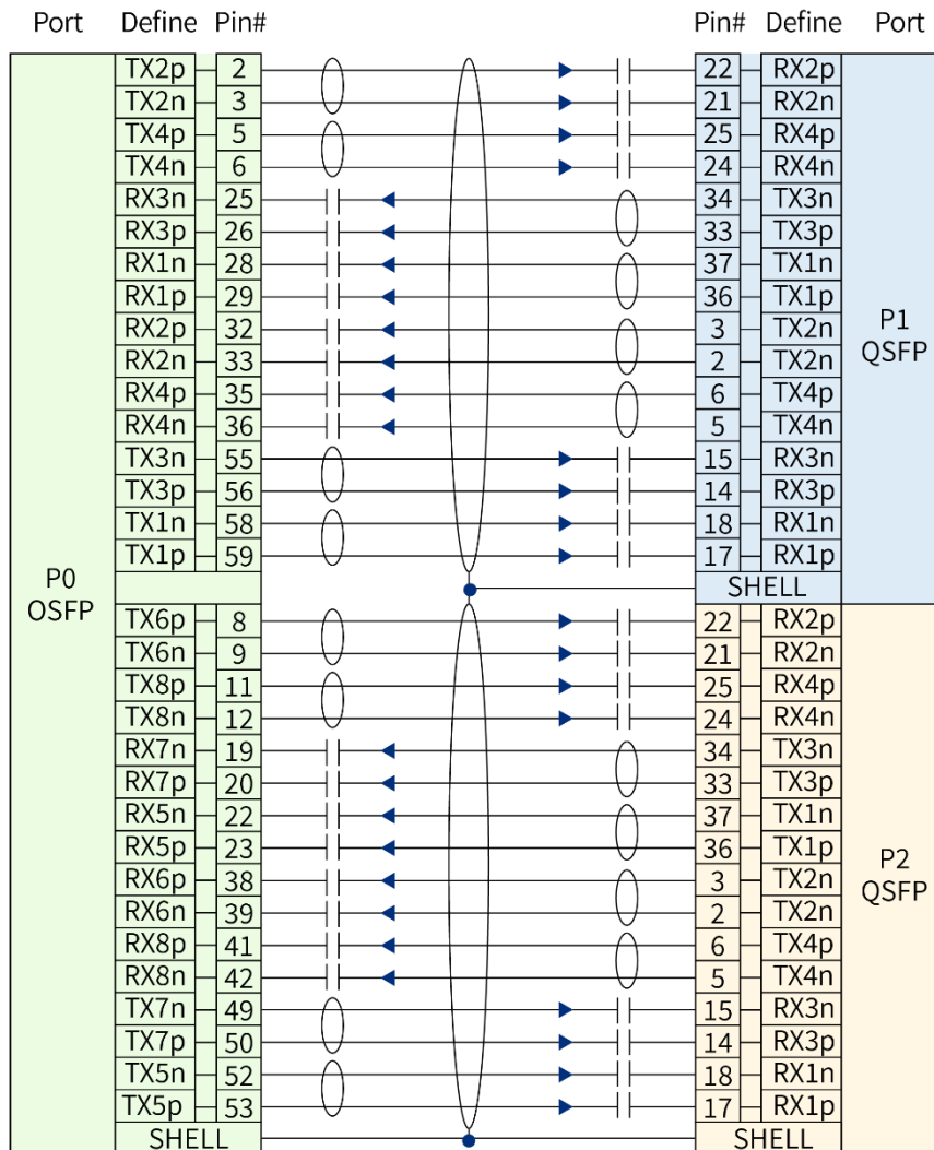
WIRING TABLE
